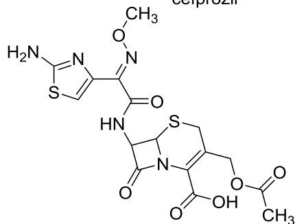
cefotaksim
