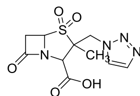
tazobaktam
