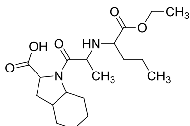
perindopril
