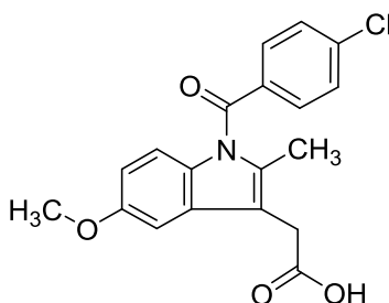
indometacin
