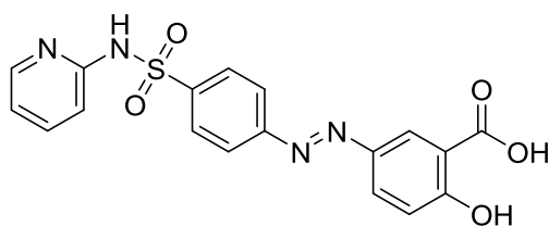
sulfasalazin
